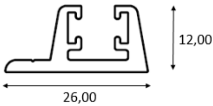
ONDERRAIL F-PROFIEL
