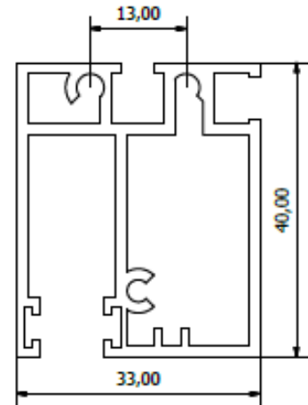
VERSTEVIGD PROFIEL (B & O)
