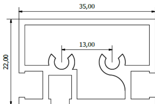
VLEUGELPROFIEL (zijkant)
