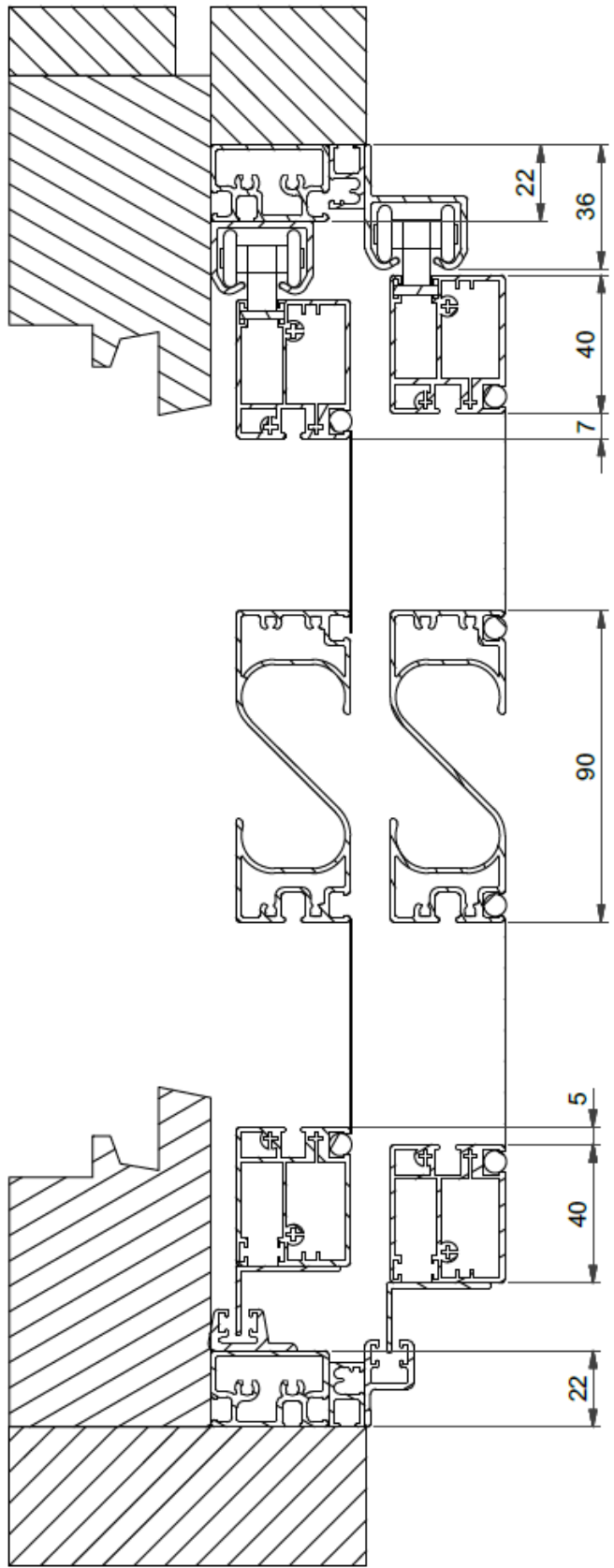
Schuifvliegendeur in en op kader
