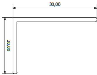
HOEK 20/30
