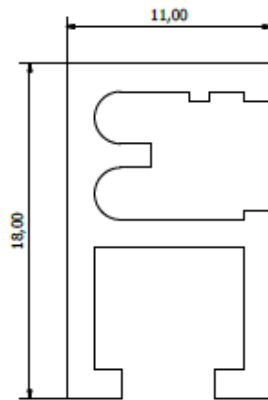
11 MM PROFIEL
